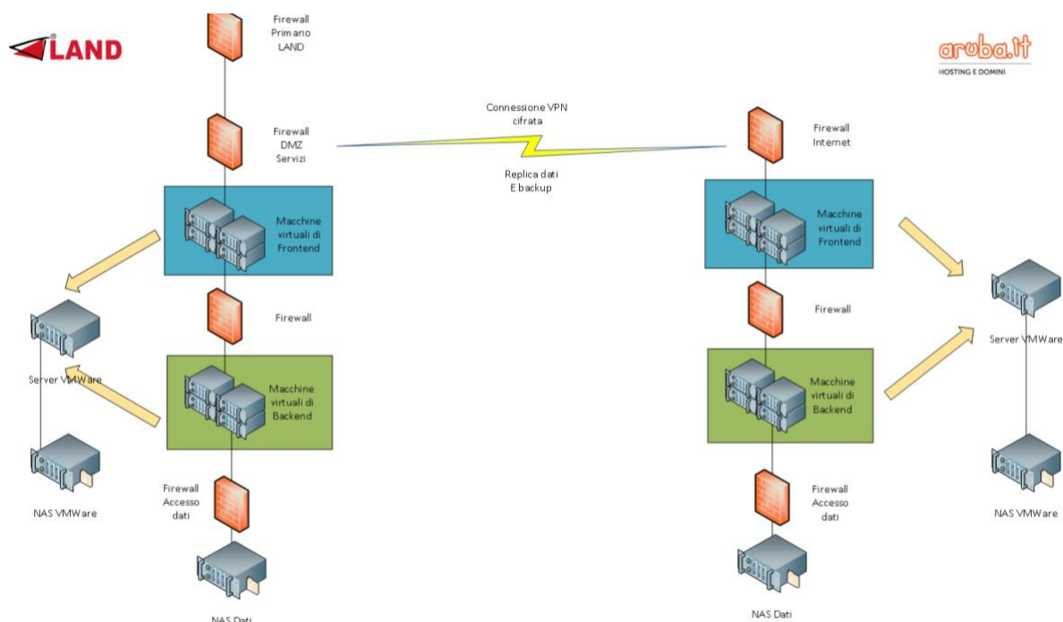
Figura 16 - Disegno dell'architettura in esercizio
